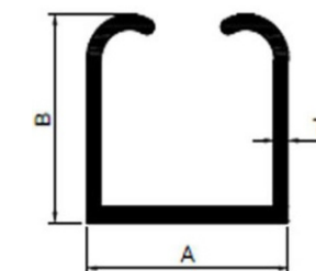
SN - 14 Door Track
